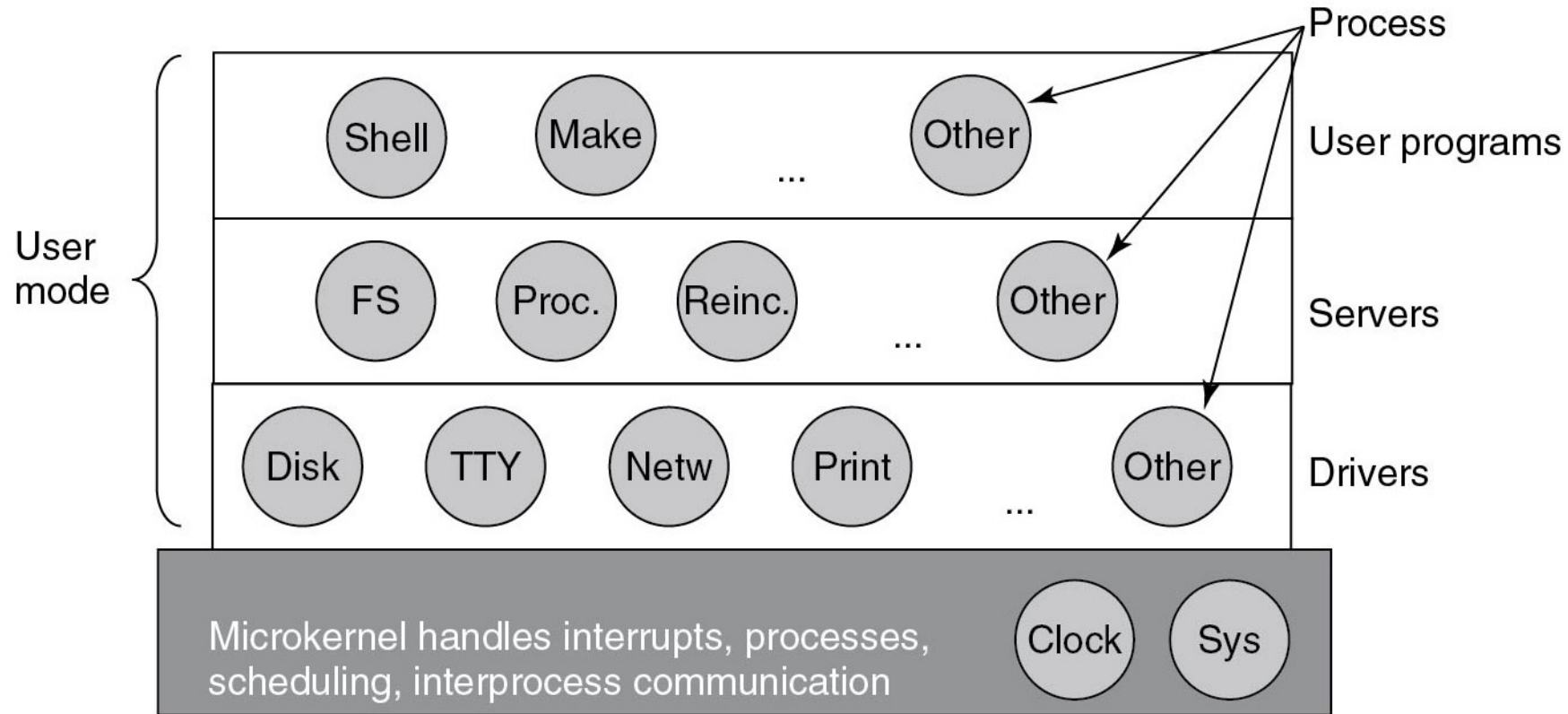
Struttura semplificata del sistema MINIX
